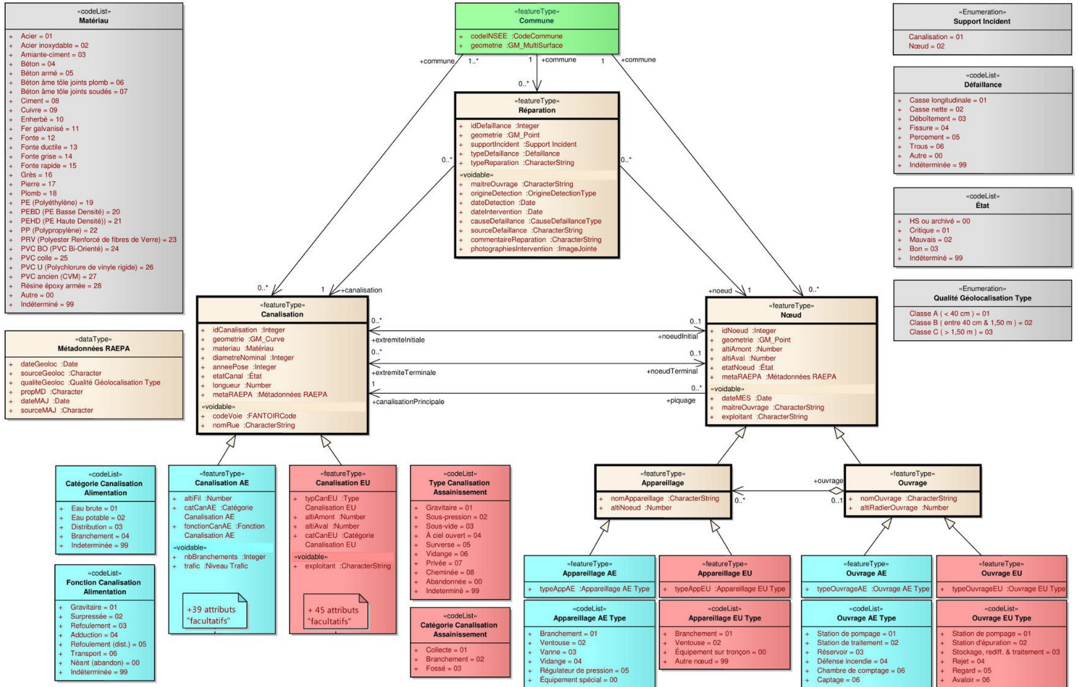
Schéma d'application UML
